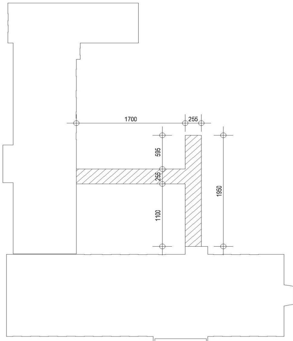
ОСНОВА ПРИЗЕМЉА - ПАСАРЕЛА - ТОПЛА ВЕЗА
