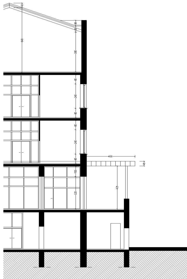
Слика 1 - Основа и пресек - постојеће стање - Надстрешница -
